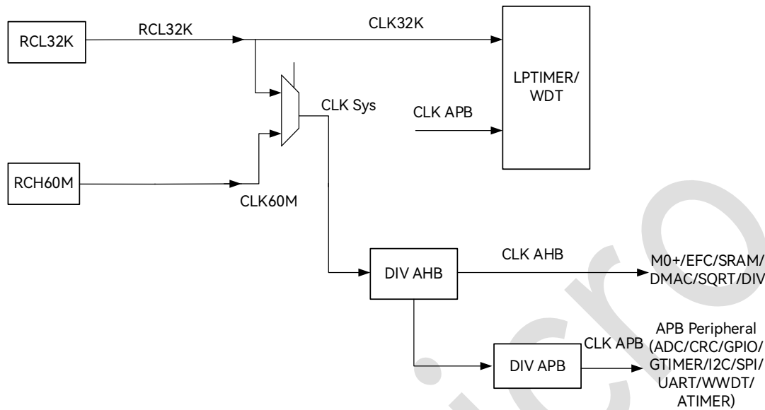
图 2-1：时钟架构图
