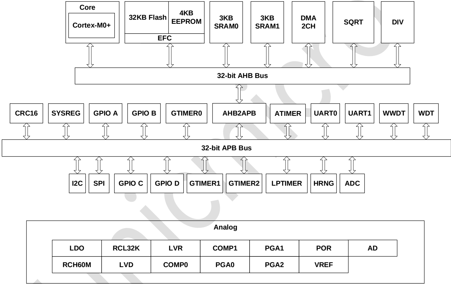
图 1-1：功能框图
