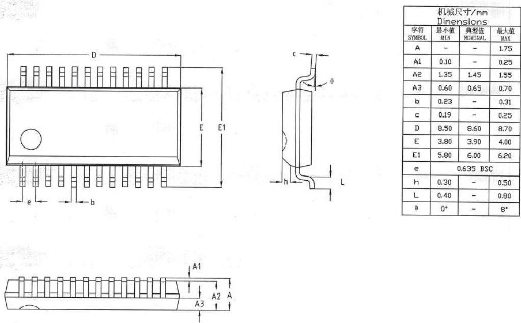
图 5-2: SSOP24 封装尺寸图
